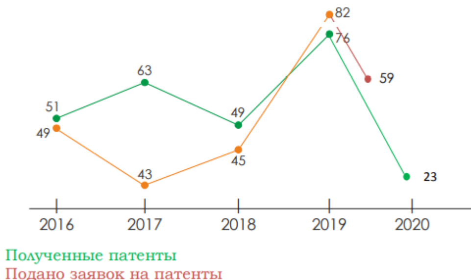
Рисунок 31 Динамика количества патентов
