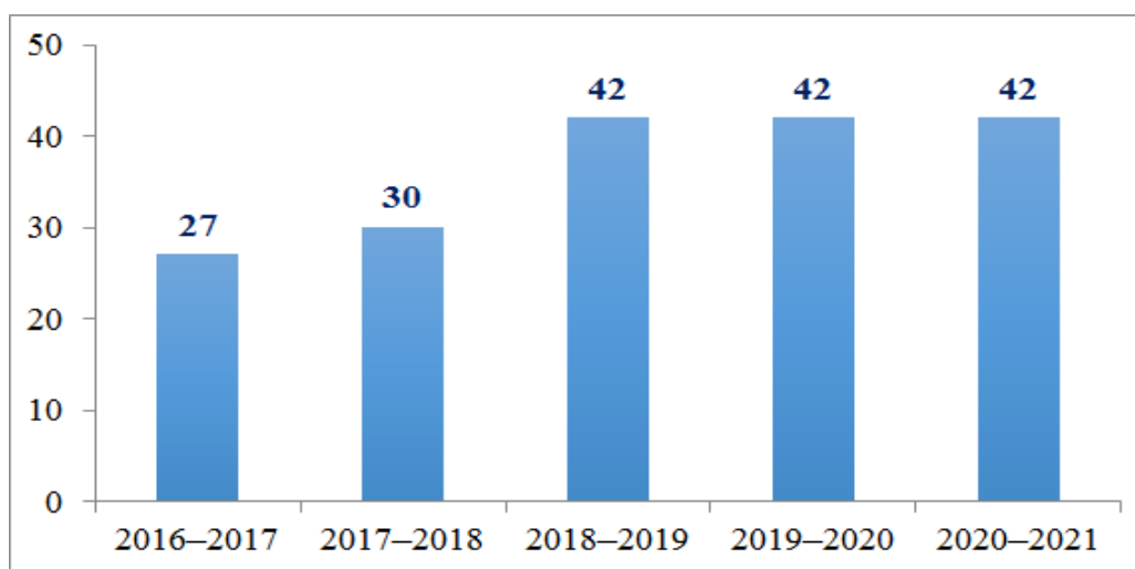
Рисунок 3 Динамика роста практико-ориентированных образовательных программ
