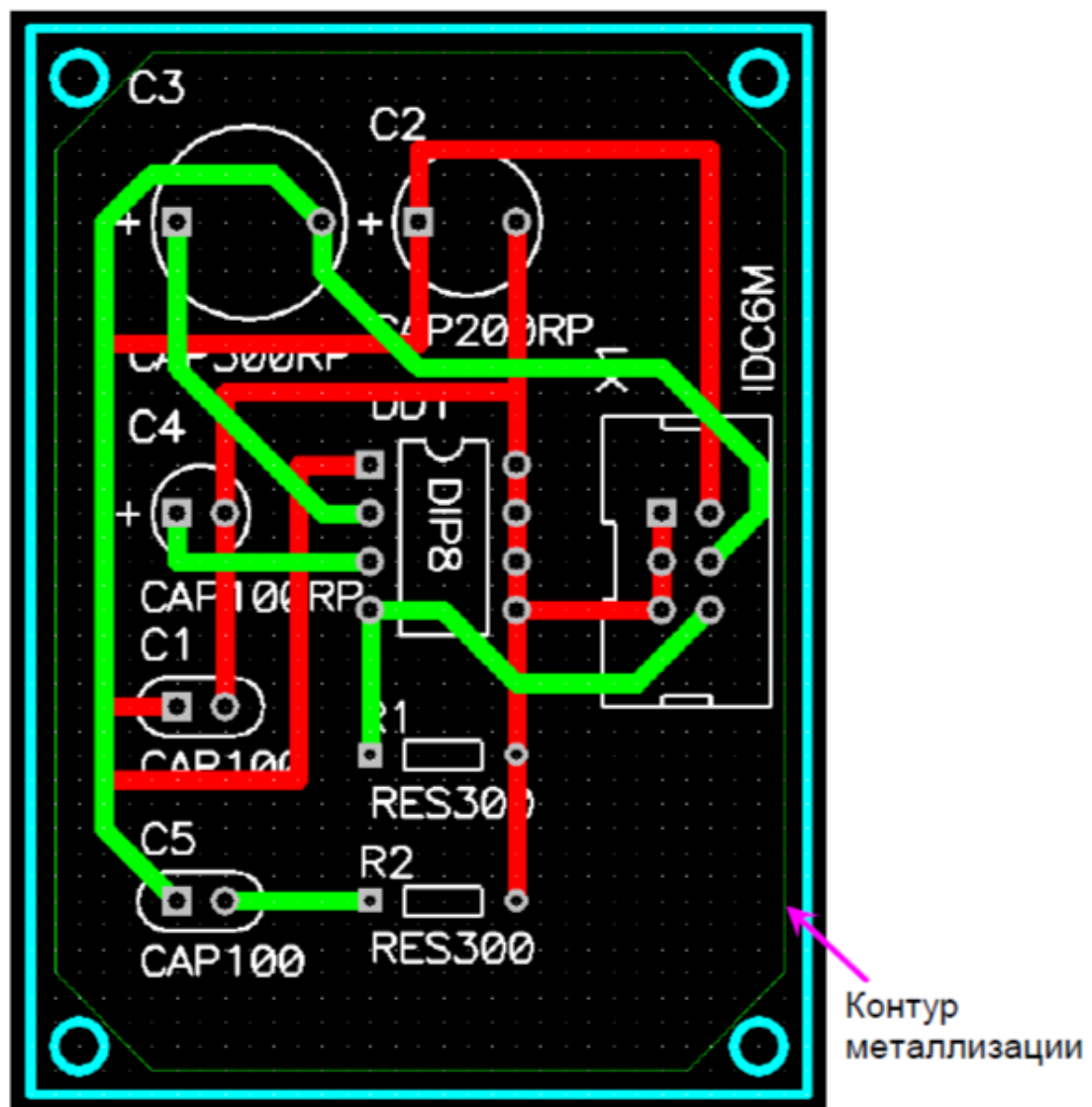
Рис. 4. Пример контура металлизации
